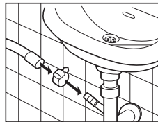
Tyhjennys poistoletkuun
